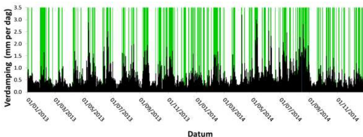
Afbeelding 1. Gemeten dagelijks verdamping in het centrum van Arnhem (zwart) in 2013 en 2014. De groene achtergrond laat dagen zien met een neerslag van 1 millimeter of meer
