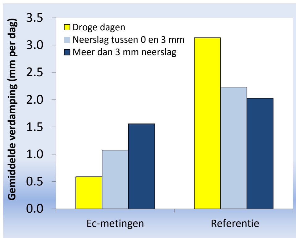
Afbeelding 2. Reactie van direct gemeten verdamping en referentieverdamping in Arnhem op neerslag
