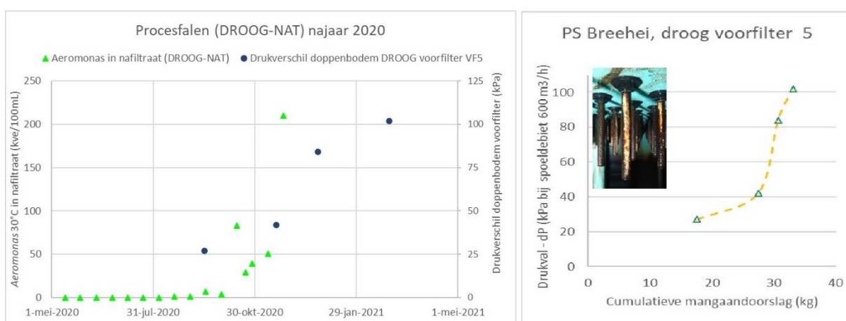
Afbeelding 5. Proces falen straat 2 (DROOG-NAT): Aeromonas in nafiltraat NF 5 en verstopping filterdoppen voorfilter VF5 (links) en relatie cumulatieve mangaandoorslag en verstopping filterdoppen in droog voorfilter VF5 (rechts)
