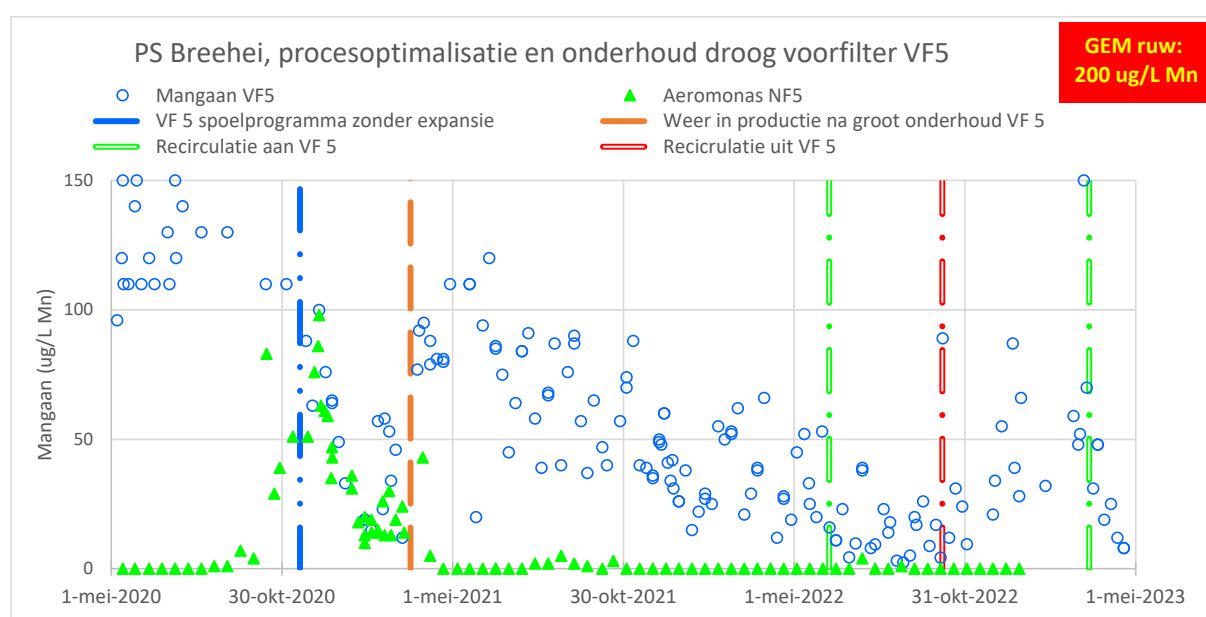
Afbeelding 6. Effecten van procesoptimalisaties en onderhoud van droog voorfilter 5 op de ontmanging in voorfilter 5 en Aeromonas in nafilts 5
