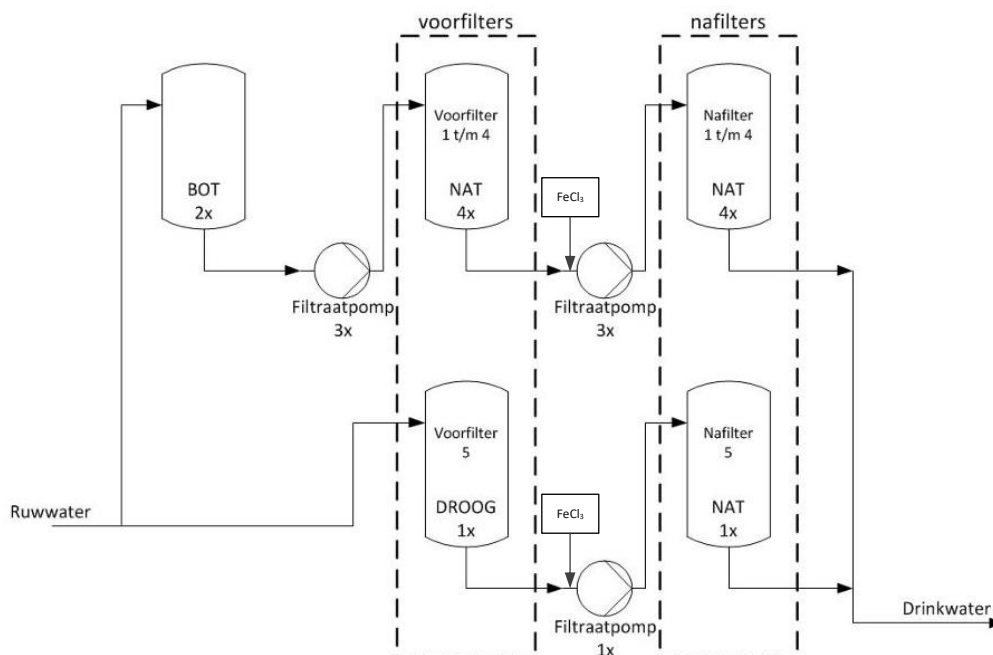
Afbeelding 1. Processchema nieuwbouw hybride zuivering PS Breehei
