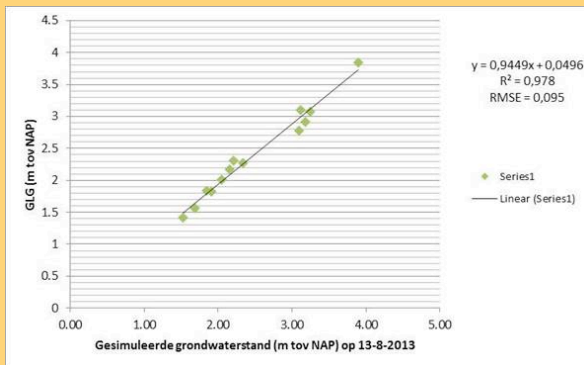
1) Regressiefiguur
